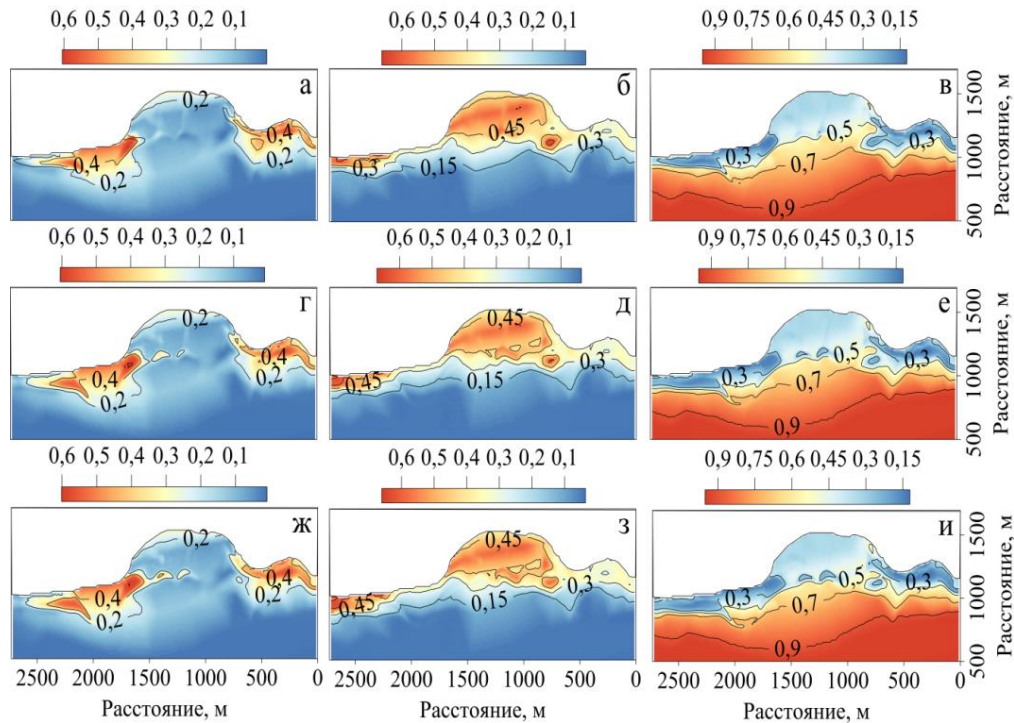
Рисунок 5 – Пространственное распределение объемных концентраций крупнозернистой (а, г, ж); среднезернистой (б, д, з); мелкозернистой (в, е, и) гранулометрических фракций при t = 12 ч для h_s = 3,6 м (а, б, в), 4,5 м (г, д, е) и 5,1 м (ж, з, и)
