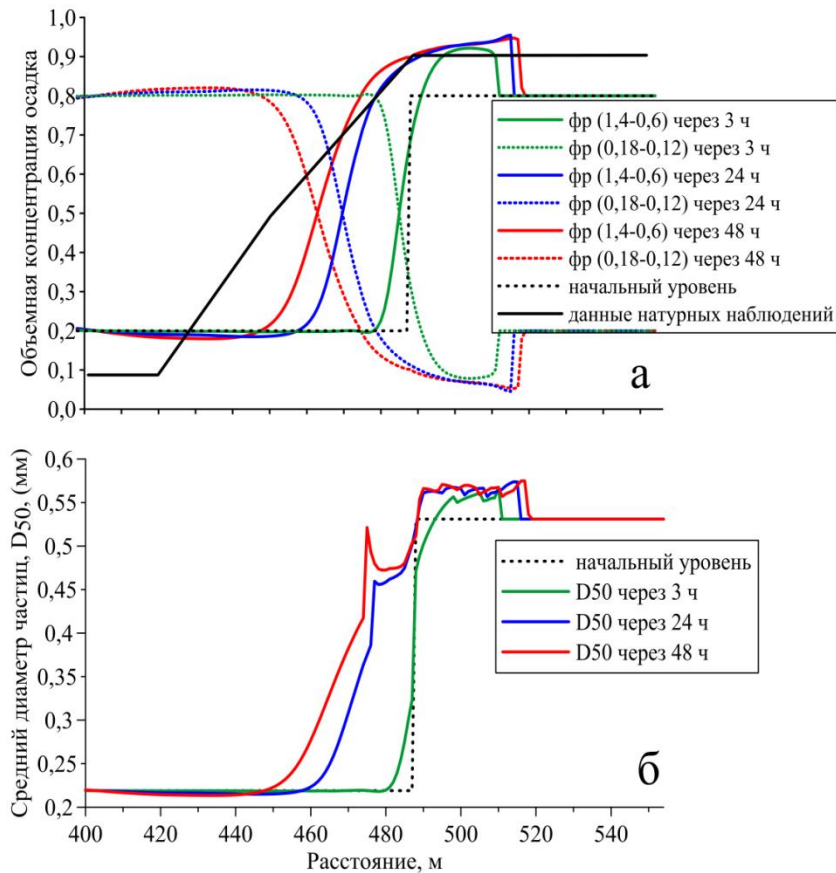
Рисунок 4 – Распределение объемных концентраций наносов (а); распределение среднего диаметра частиц ( D_{50} ) (б) для профиля BC2 (состоящего из разных по крупности наносов, разделенных на две области) ( h_s = 2 м, \tau_p = 8 )
