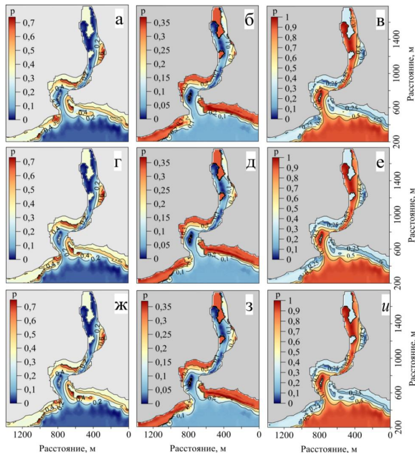
Рисунок 7 – Пространственное распределение объемных концентраций крупнозернистой (а, г, ж); среднезернистой (б, д, з); мелкозернистой (в, е, и) фракций при t = 12 ч для волнения юго-юго-восточного (а, б, в), южного (г, д, е) и юго-юго-западного (ж, з, и) направлений [11]
