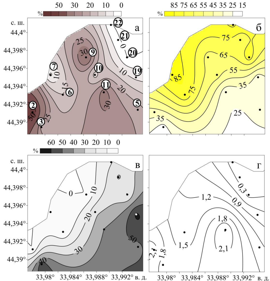
Рисунок 2 – Пространственное распределение гравийной (а), песчаной (б), алеврито-пелитовой (в) фракций и среднего диаметра частиц, мм (г) в поверхностном слое донных наносов Лименского залива; цифрами в кружочках показаны номера станций отбора проб [3]
