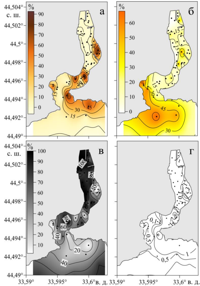
Рисунок 3 – Пространственное распределение гравийной (а), песчаной (б), илистой (в) фракций и среднего диаметра частиц, мм (г) в поверхностном слое донных наносов Балаклавской бухты в 2005–2019 гг.
