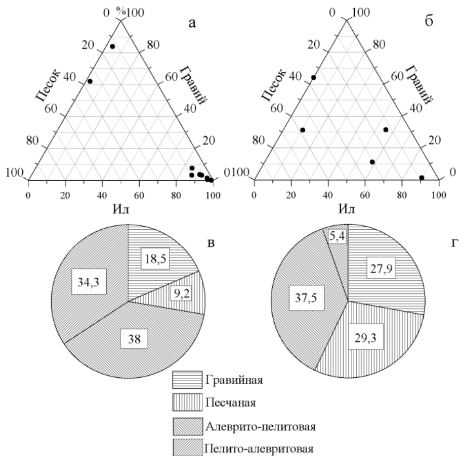
Рисунок 1 – Трехкомпонентная (а, б) и круговая (в, г) диаграммы фракционного состава донных наносов Каламитского залива в 2011 (а, в) и 2012 (б, г) гг.
