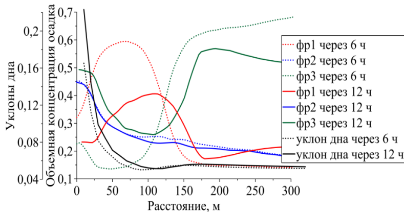
Рисунок 6 – Особенности перераспределения гранулометрических фракций и динамика угла наклона дна для южного волнения, h_s = 5 м
